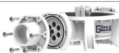
Retirez les 6 vis retenant la bride au corps de la pompe.
