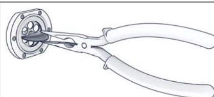
Utilisez des pinces pour retirer l'ancienne valve parapluie de la butée de valve.
